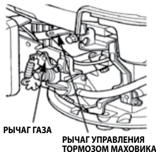
ТИП 1: ТОРМОЗ МАХОВИКА/ ДИСТАНЦИОННЫЙ ДРОССЕЛЬ
