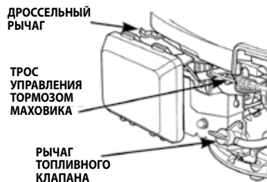
ТИП 4: АВТОМАТИЧЕСКИЙ ВОЗВРАТ ДРОССЕЛЯ/ ФИКСИРОВАННЫЙ ГАЗ
