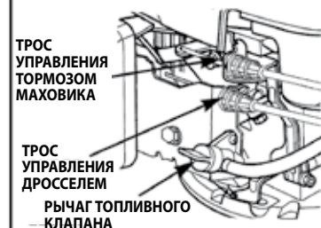
ТИП 3: ТОРМОЗ МАХОВИКА/ ДИСТАНЦИОННЫЙ ДРОССЕЛЬ/ ФИКСИРОВАННЫЙ ГАЗ
