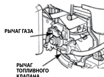
ТИП 6: ДИСТАНЦИОННЫЙ ДРОССЕЛЬ/ СЦЕПЛЕНИЕ ТОРМОЗА ЛОПАСТИ (управление оборудованием)
